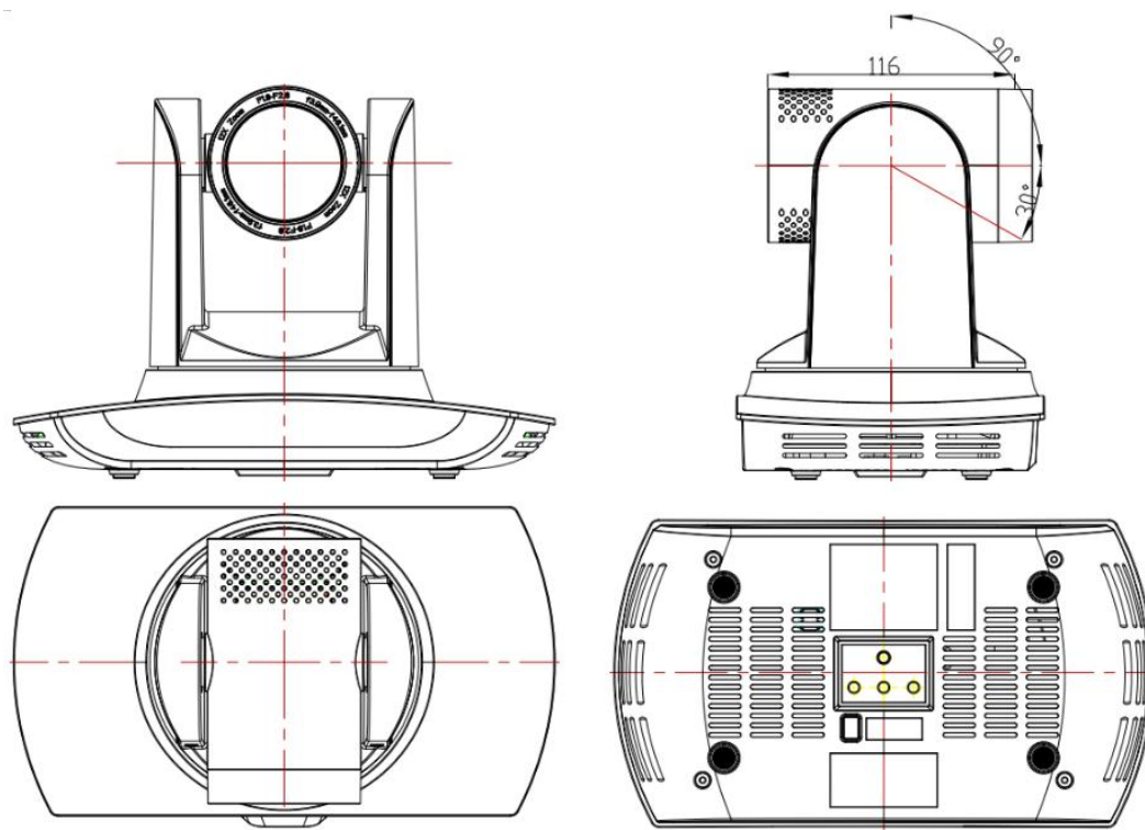
図2.2 製品寸法
