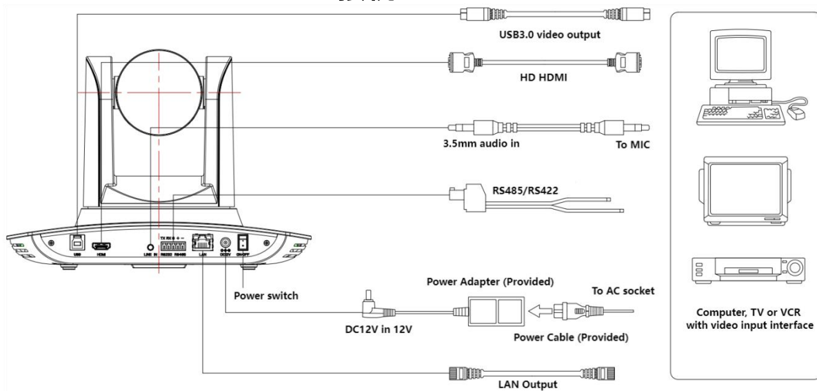
図1.2 配線図
